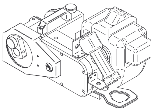
Figura 3 : Verricello completo
