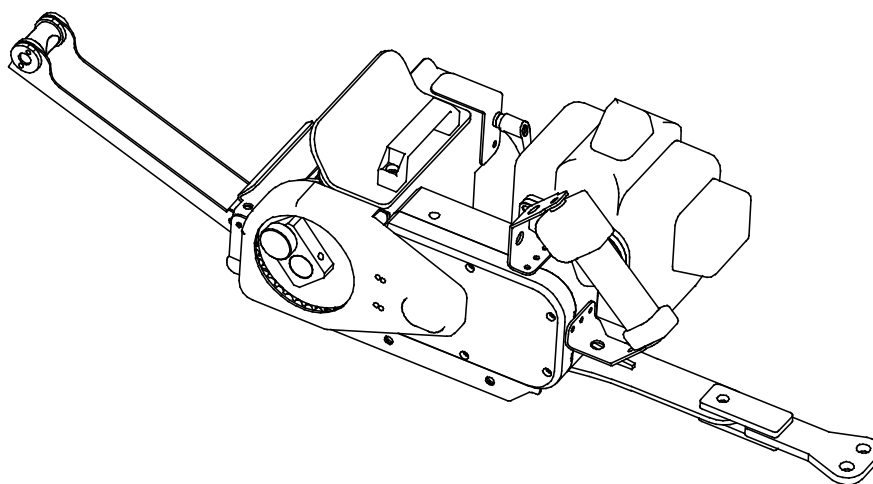
Figura 3 : Verricello completo
