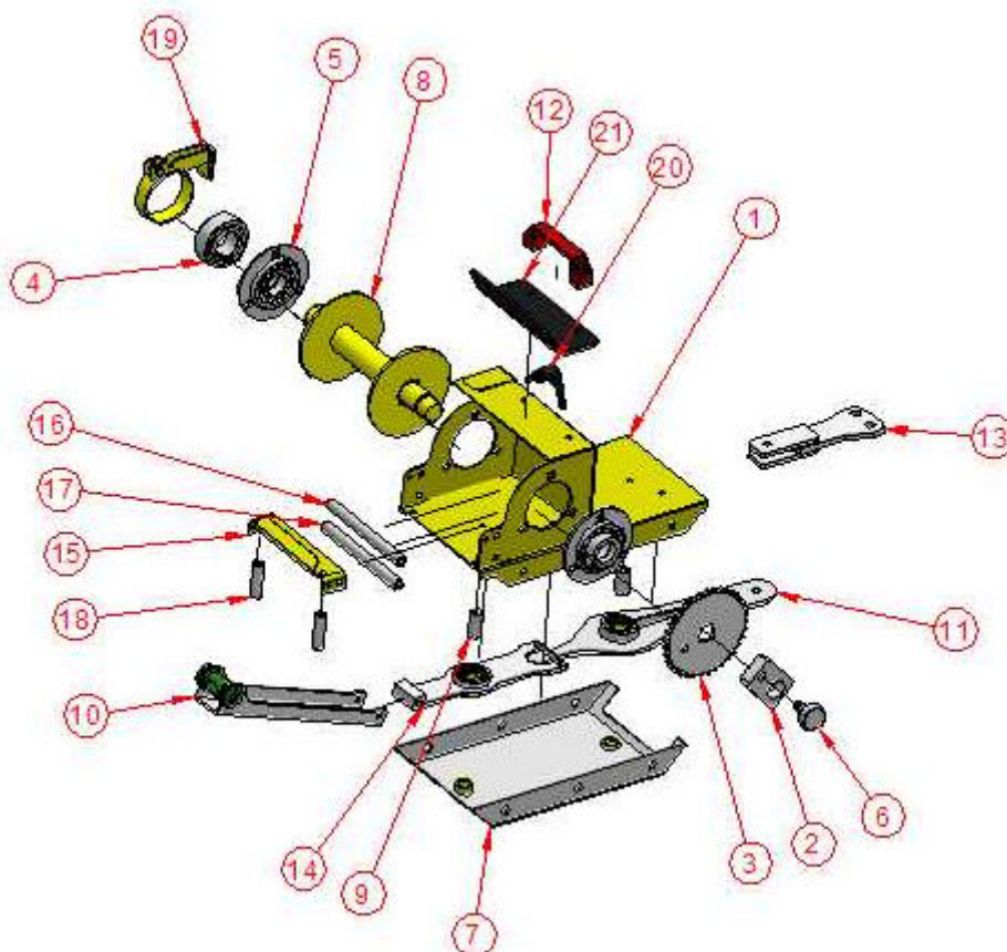
Figura 2 : Vista esplosa del gruppo telaio
